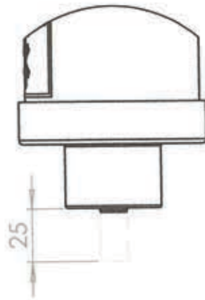
Detalhe A Pino Percursor 12kgf
