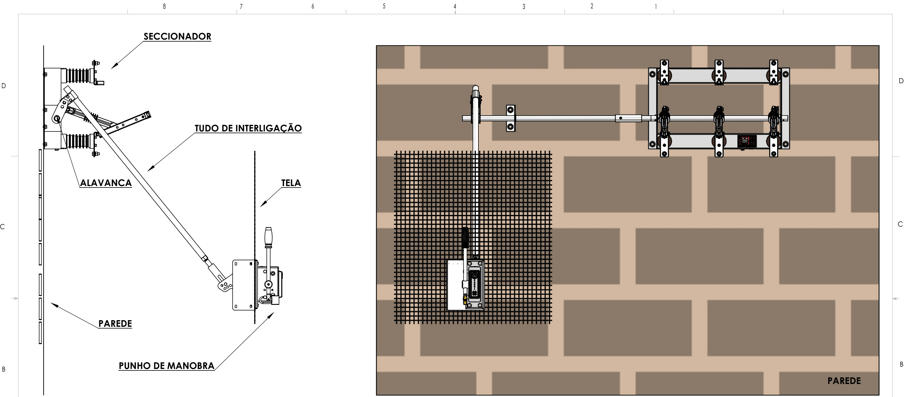
VISTA FRONTAL DA INSTALAÇÃO OPERADOR DE FRENTE PARA OPERAÇÃO
